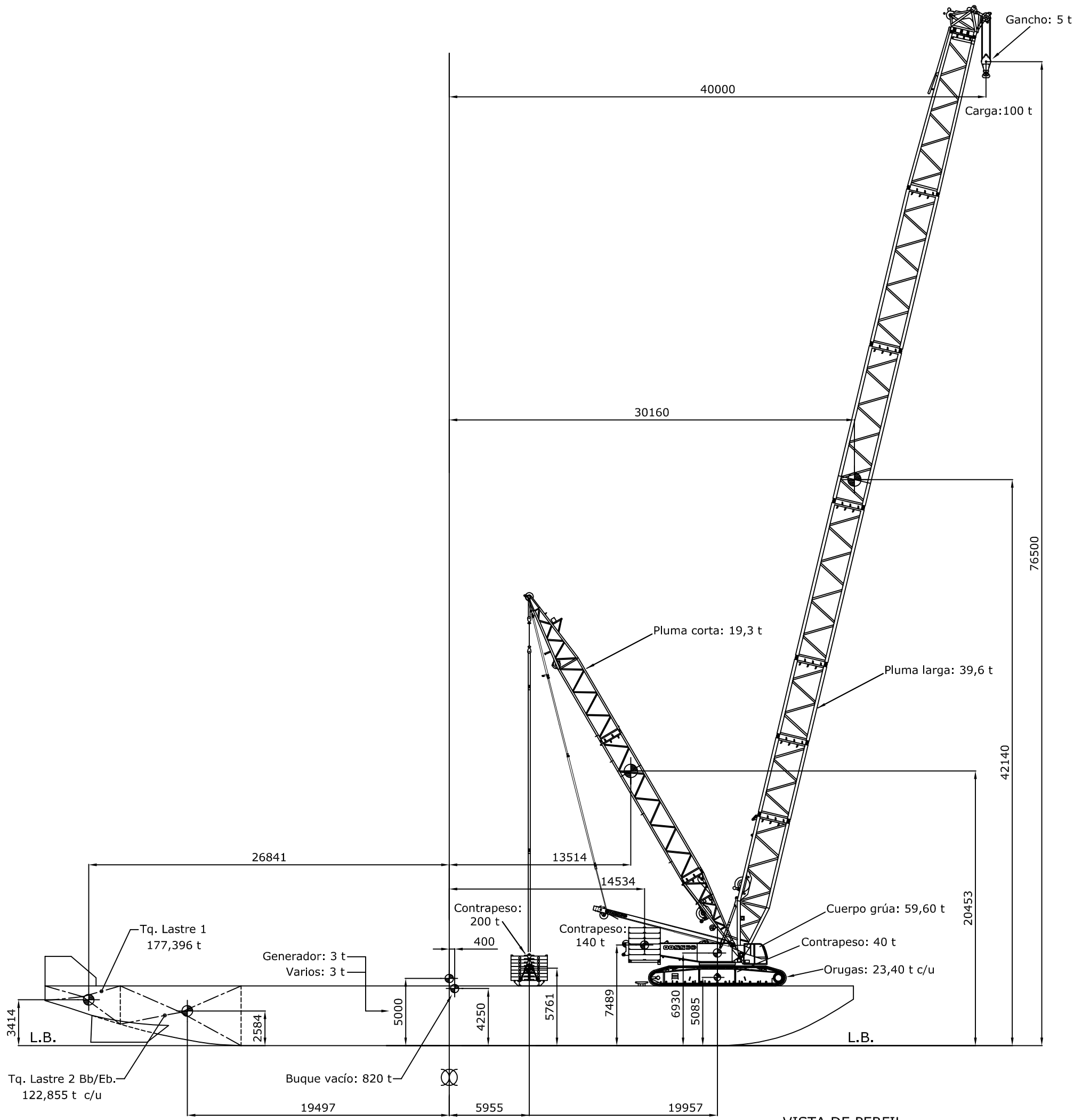
VISTA DE PERFIL
